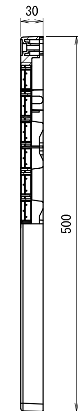
断面 A-A 水抜き穴用ノック
