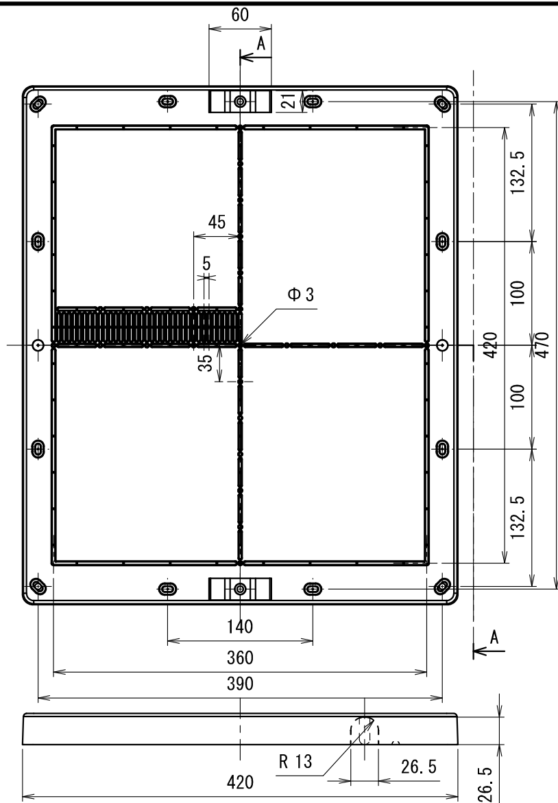
断面 A-A 水抜き穴用ノック
